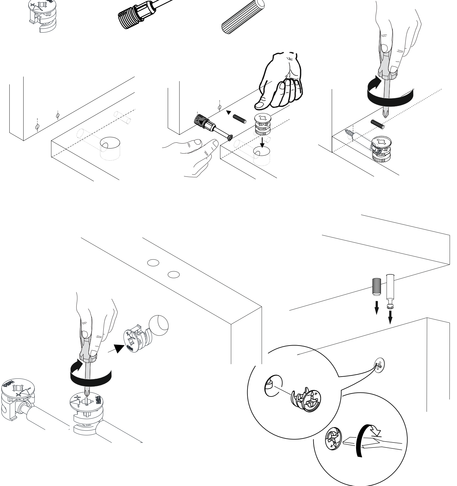
Minifix Gövde
